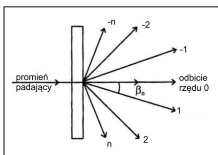
siatka dyfrakcyjna transmisyjna
