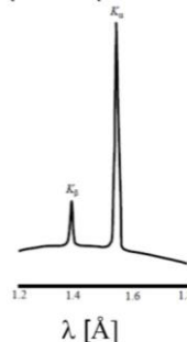
widmo promieniowania lampy rentgenowskiej z anodą miedzianą
